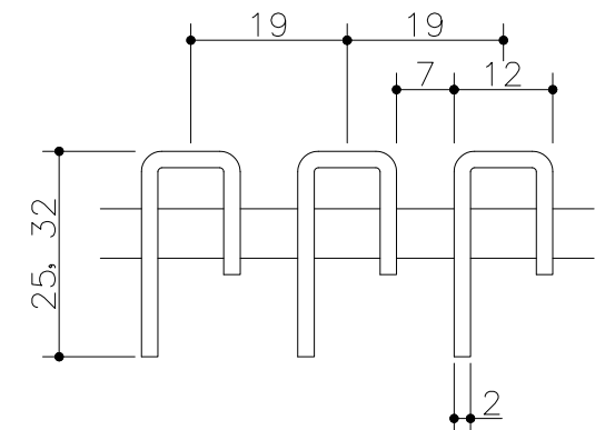
Jバー断面詳細図
