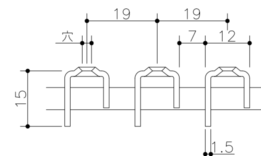
Jバー断面詳細図
