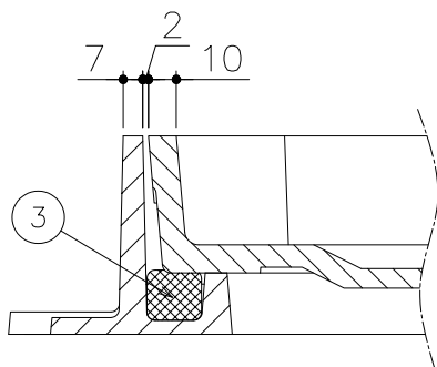
目地部詳細
