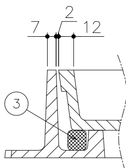
目地部詳細
