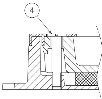
ボルト固定部詳細
