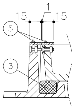
目地部詳細
