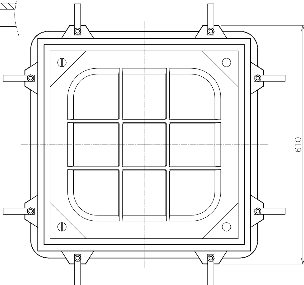
ボルト固定部詳細
