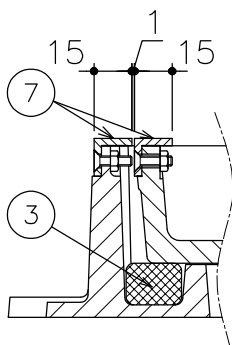
目地部詳細
