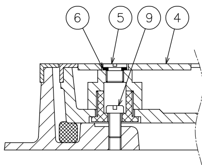
ボルト固定部詳細
