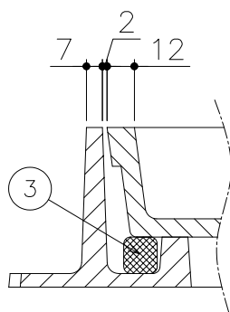
目地部詳細
