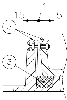
目地部詳細
