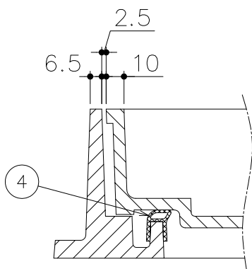
詳細図
