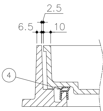
詳細図
