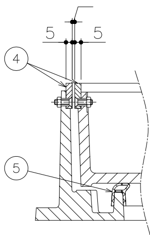
目地部詳細
