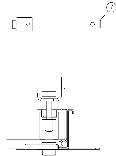
蓋開閉方法
