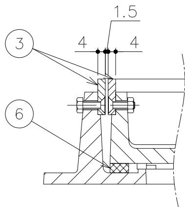
目地部詳細
