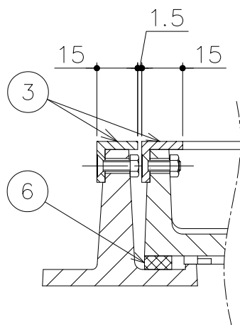
目地部詳細
