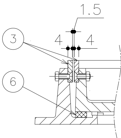
目地部詳細
