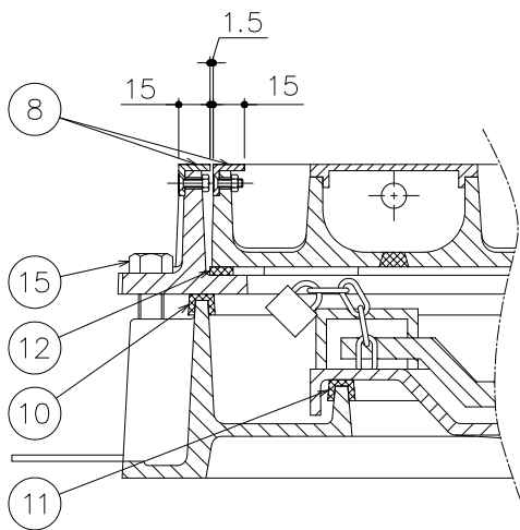
目地部詳細
