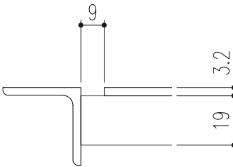
A部詳細図 S=1/2
