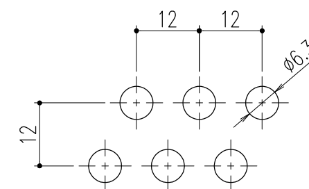
底面 排水穴形状 S=1/1
