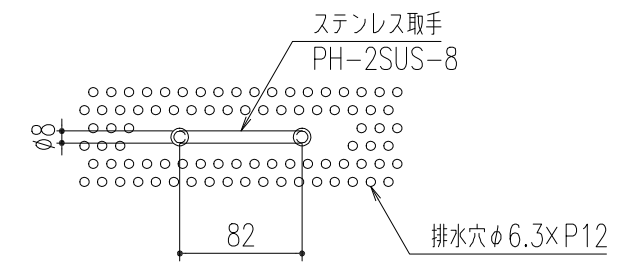
バスケット詳細図
