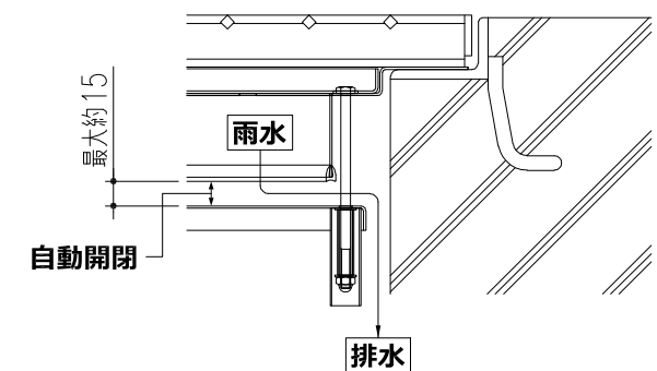
開閉時状態図
