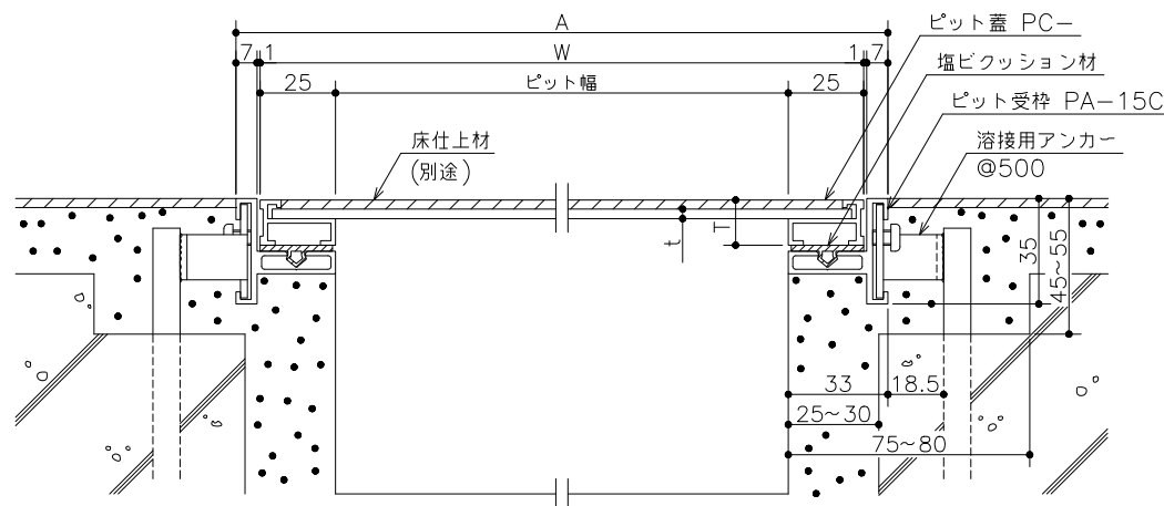
断面詳細図 S=1/2
