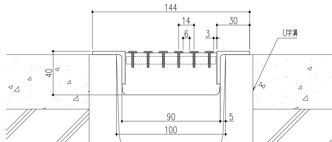
断面詳細図 S=1/2
