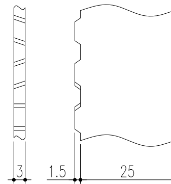
ベアリングバー詳細図
