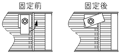
グレーチング固定部詳細図
