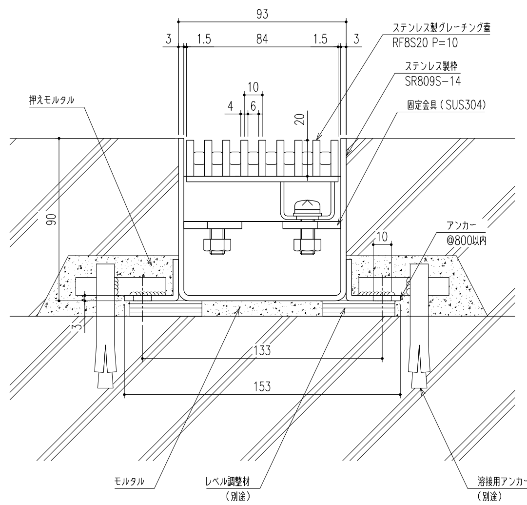
断面詳細図 S=1/2 【溶接固定納まり】
