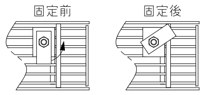
グレーチング固定部詳細図
