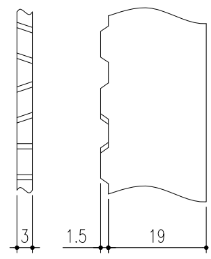
ベアリングバー詳細図
