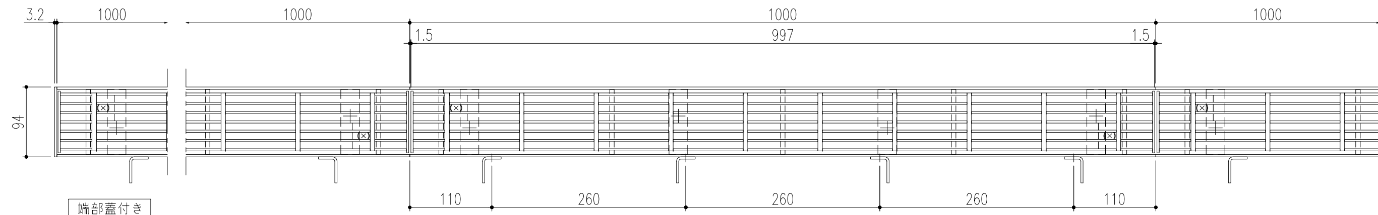
平面詳細図 S=1/5
