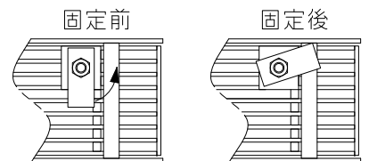
グレーチング固定部詳細図
