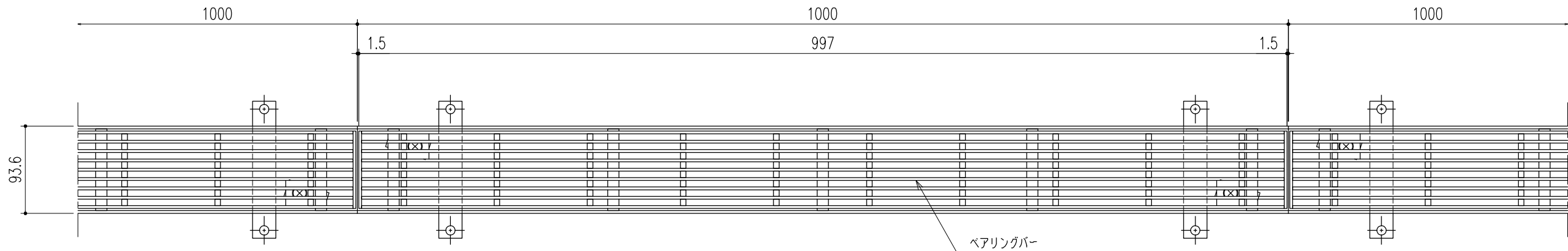
平面詳細図 S=1/5
