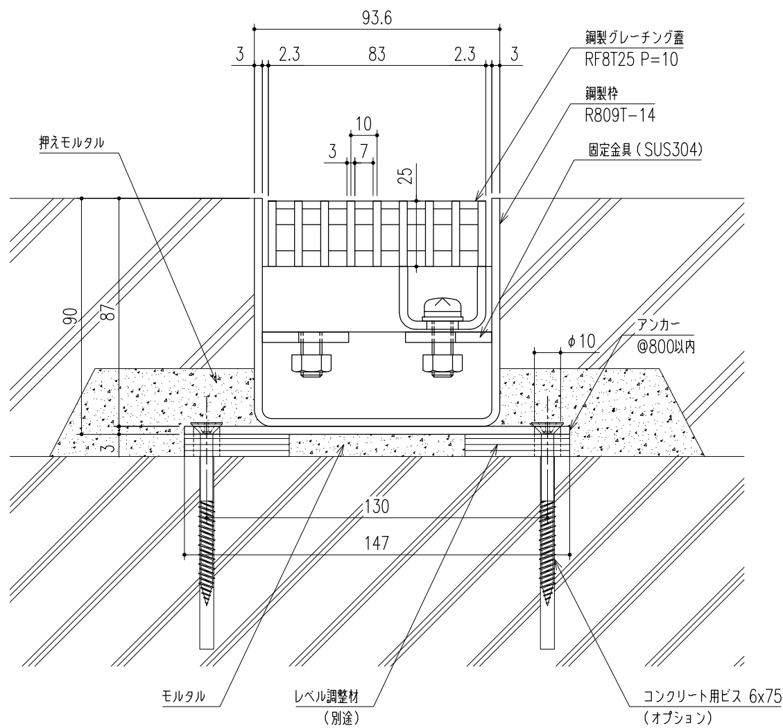
断面詳細図 S=1/2 【コンクリート用ビス固定納まり】
