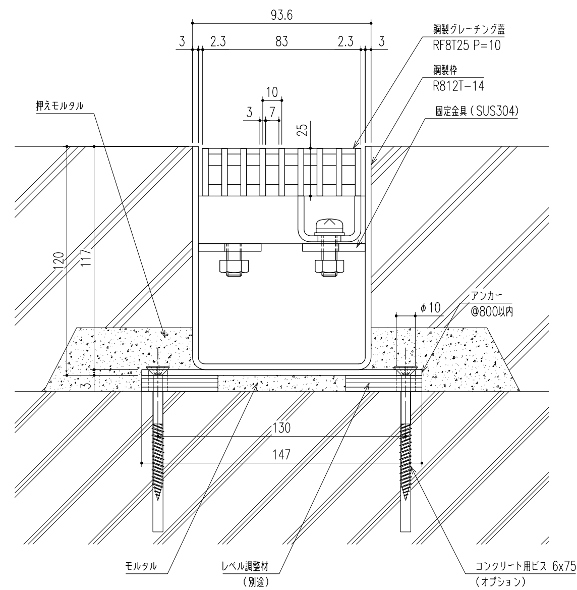
断面詳細図 S=1/2 【コンクリート用ビス固定納まり】
