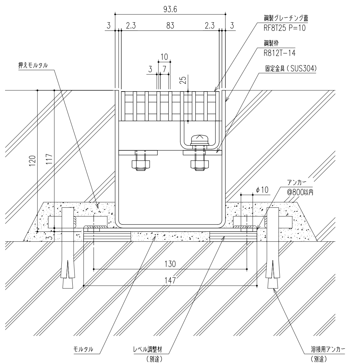
断面詳細図 S=1/2 【溶接固定納まり】
