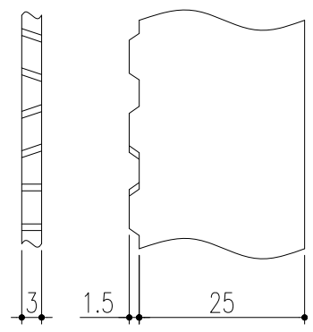
ベアリングバー詳細図
