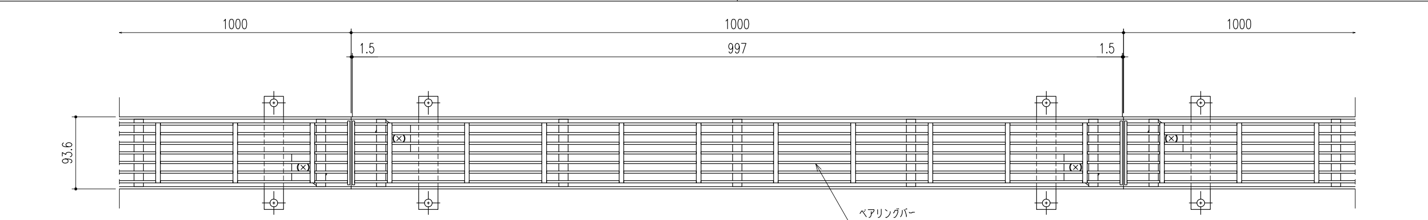
平面詳細図 S=1/5
