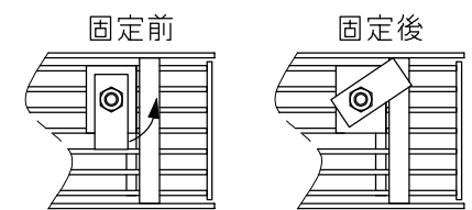
グレーチング固定部詳細図
