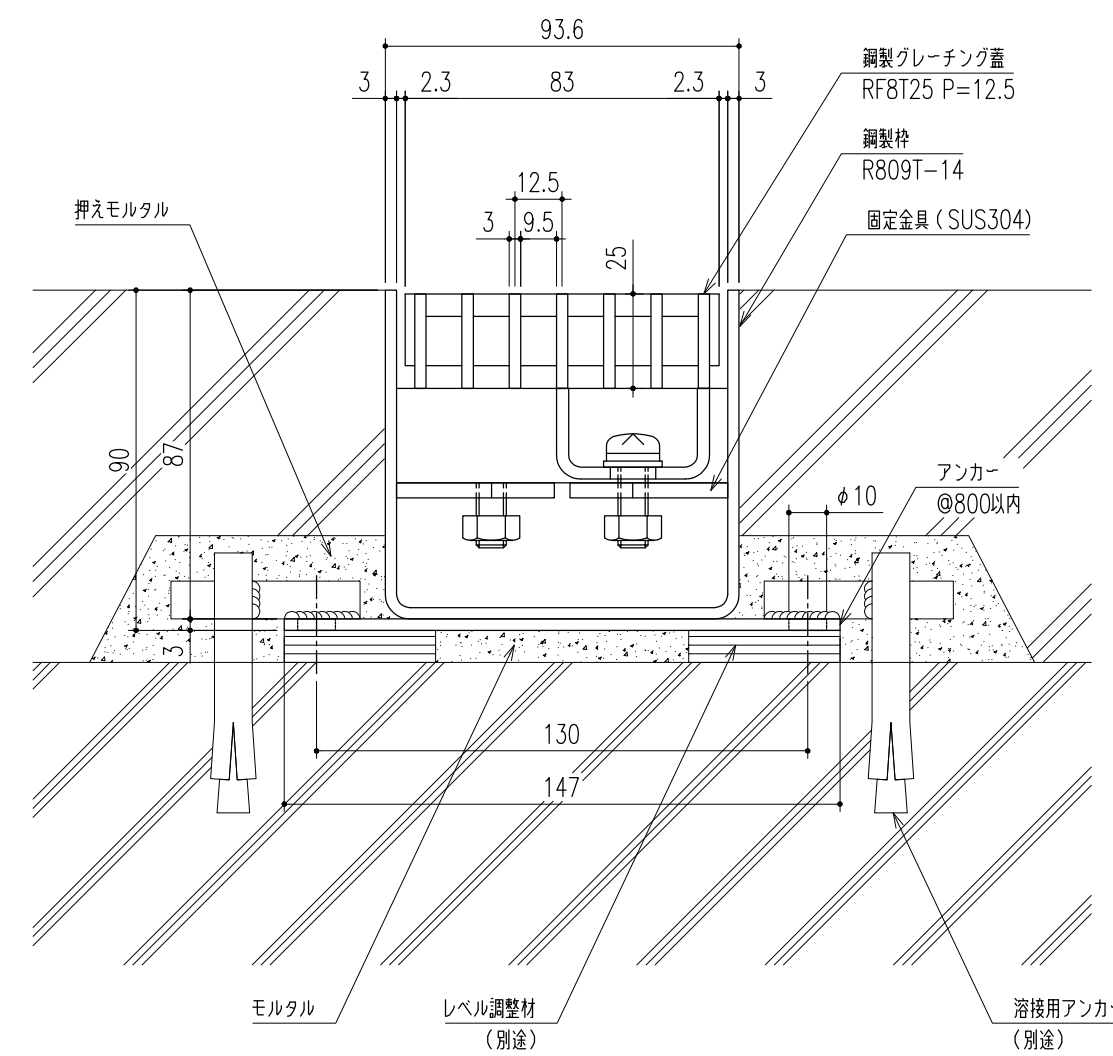
断面詳細図 S=1/2 【溶接固定納まり】
