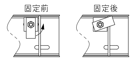
蓋固定部詳細図
