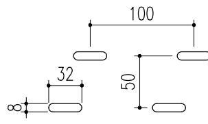
蓋排水穴形状
