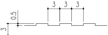
蓋断面詳細図
