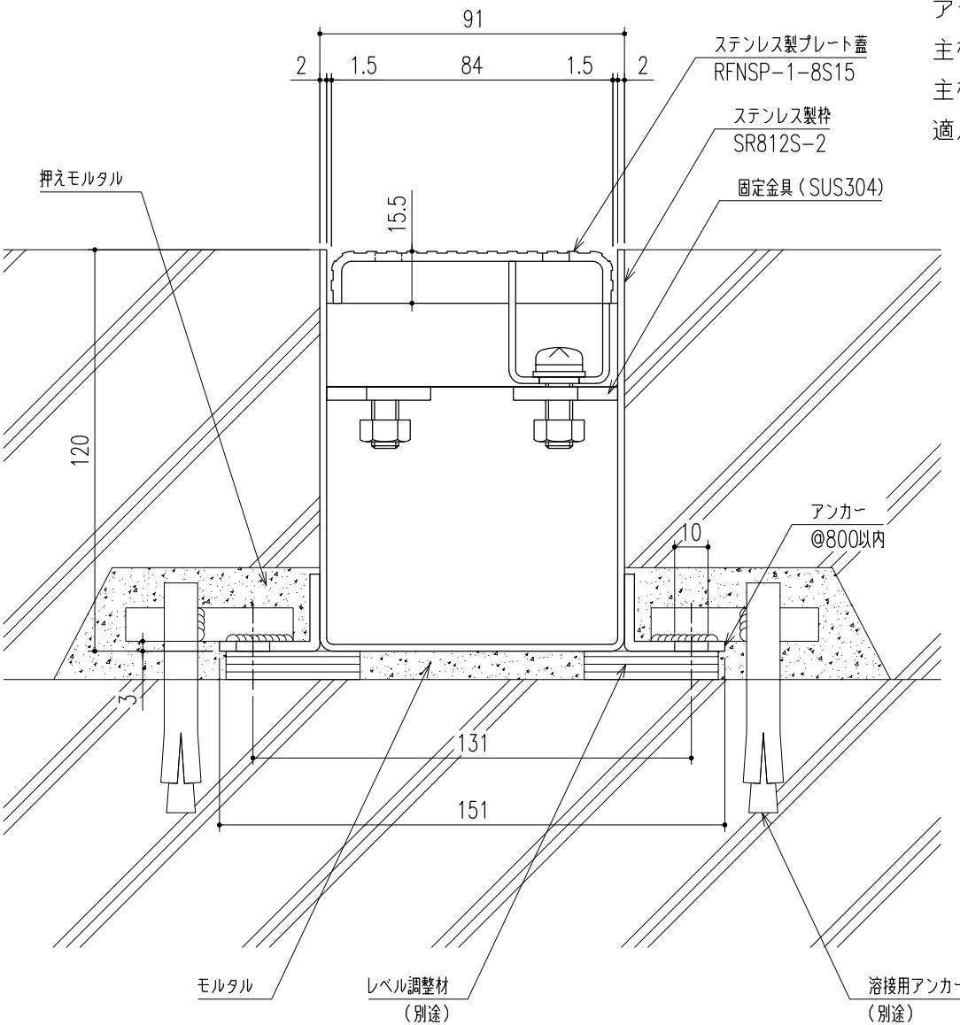
断面詳細図 S=1/2
