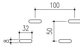
蓋排水穴形状
