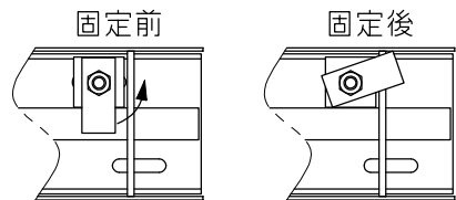
蓋固定部詳細図
