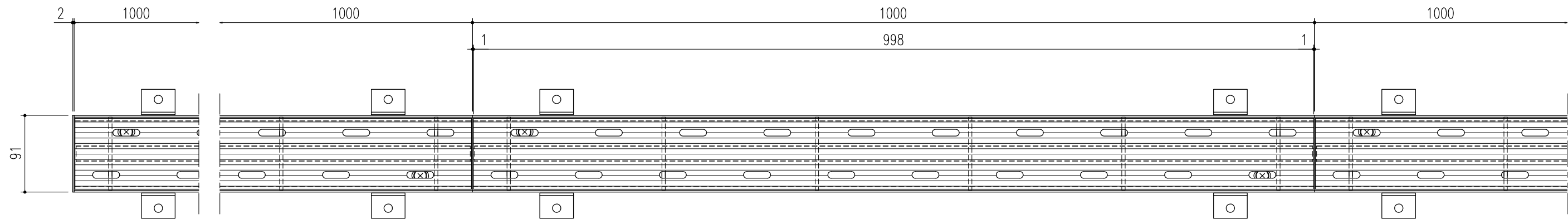
端部蓋付き
