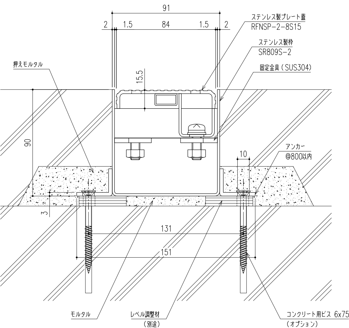
端部蓋付き
