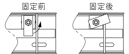
蓋固定部詳細図
