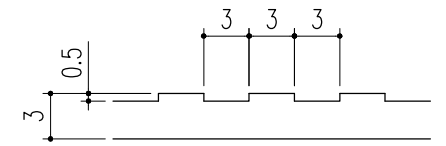
蓋断面詳細図
