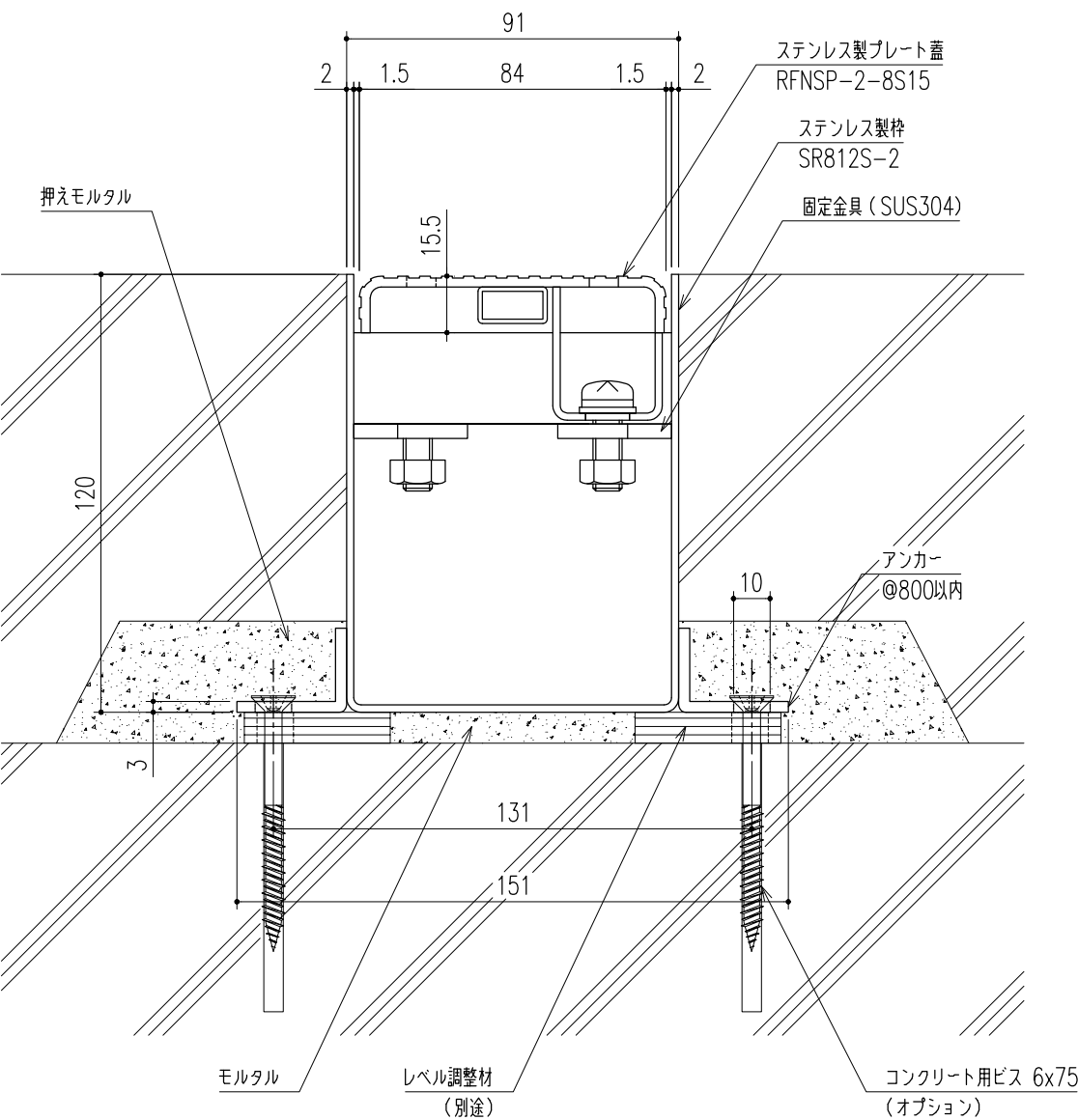
断面詳細図 S=1/2
