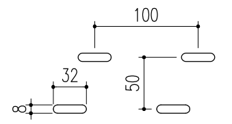
蓋排水穴形状
