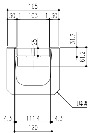
断面詳細図
