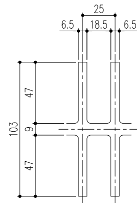
排水部詳細図 S=1/2
