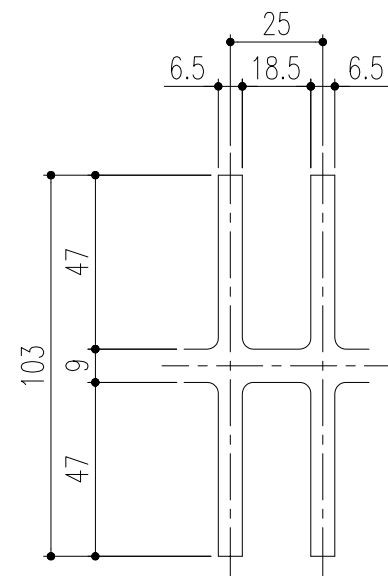
排水部詳細図 S=1/2
