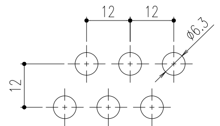
排水穴詳細図 S=1/1
