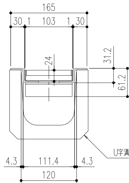
断面詳細図
