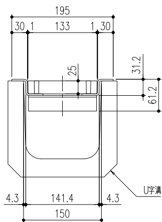
断面詳細図
