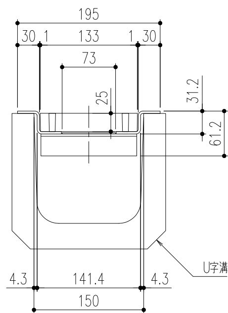
断面詳細図
