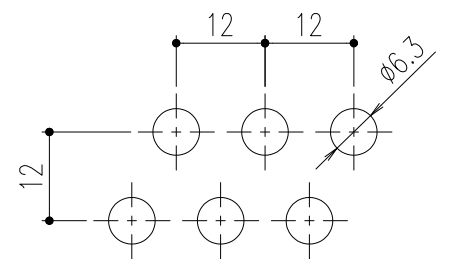
排水穴詳細図 S=1/1
