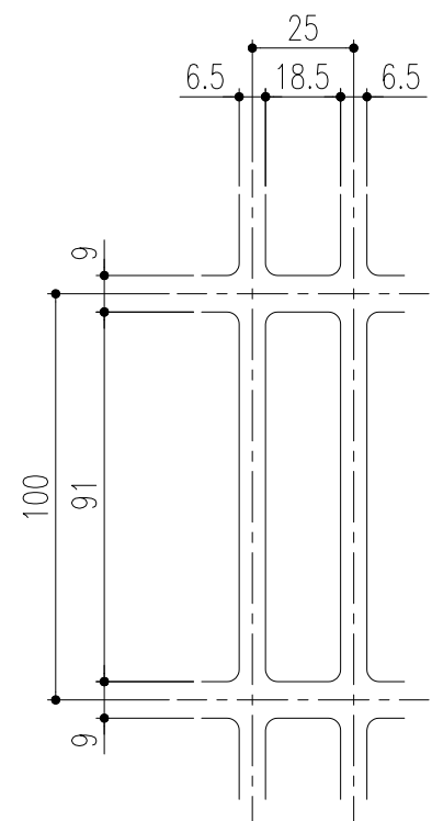
排水部詳細図 S=1/2
