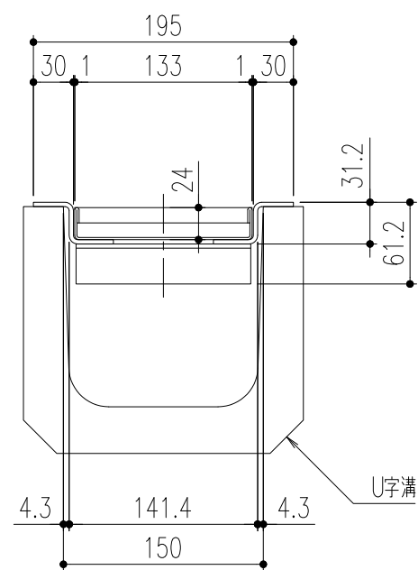
断面詳細図
