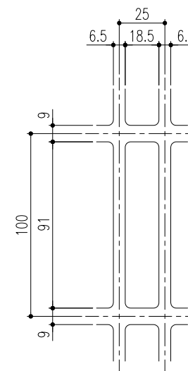
排水部詳細図 S=1/2
