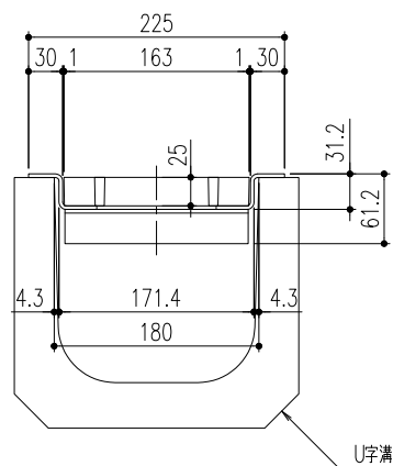
断面詳細図
