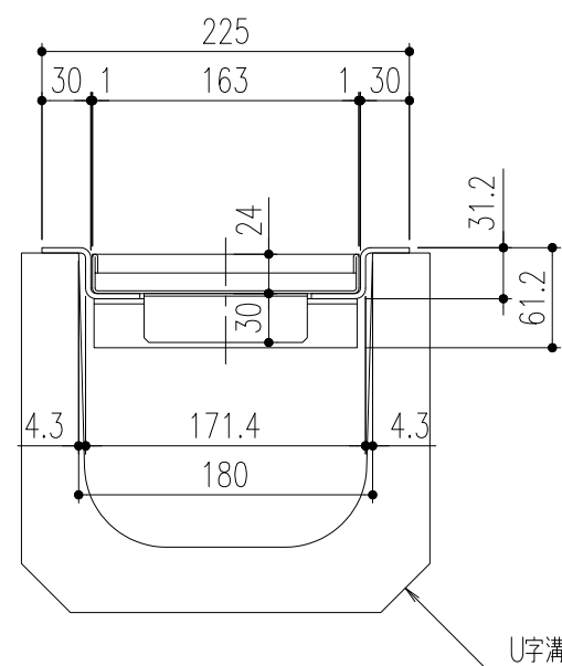
断面詳細図
