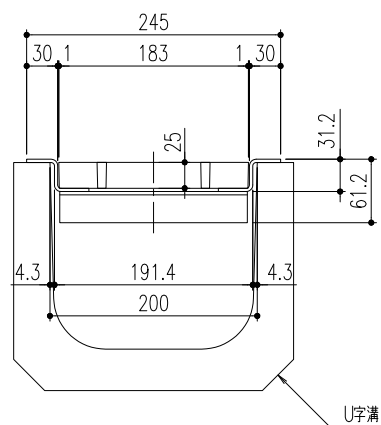
断面詳細図
