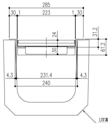
断面詳細図
