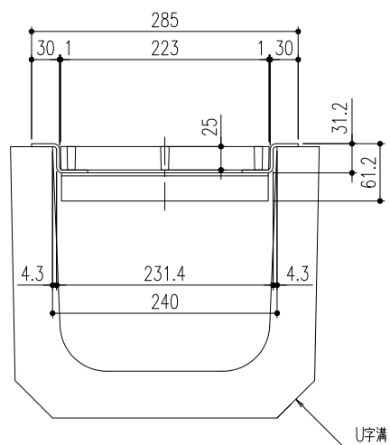
断面詳細図
