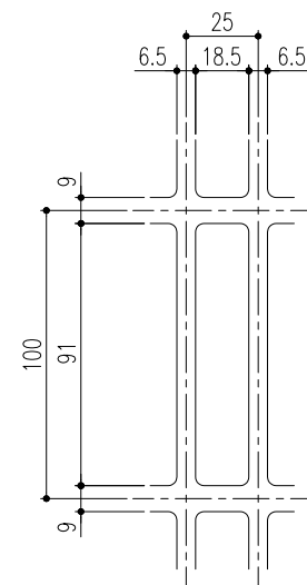
排水部詳細図 S=1/2
