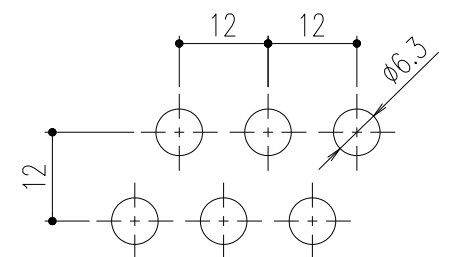
排水穴詳細図 S=1/1
