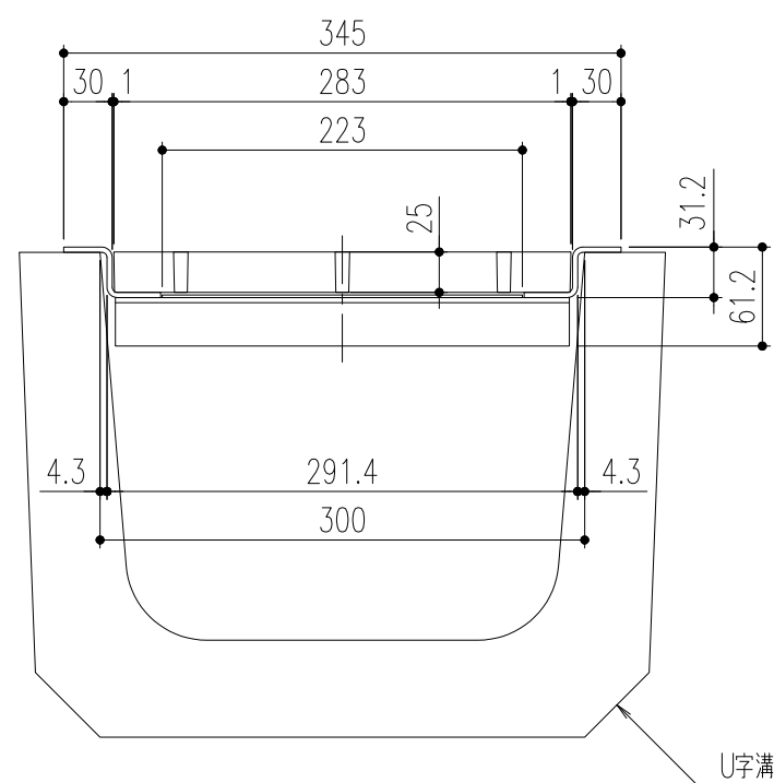
断面詳細図
