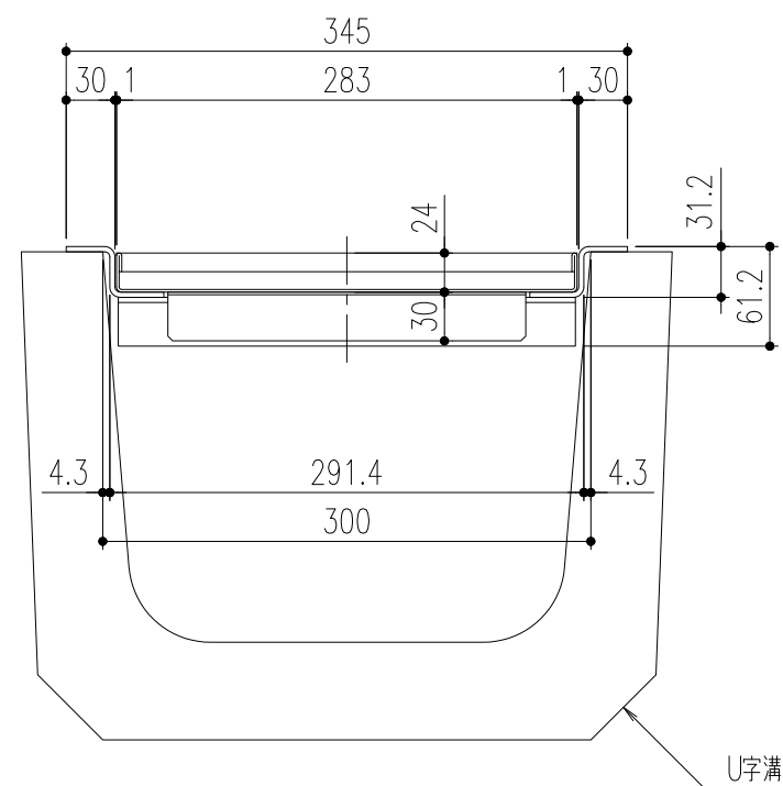
断面詳細図
