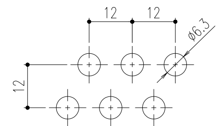
排水穴詳細図 S=1/1
