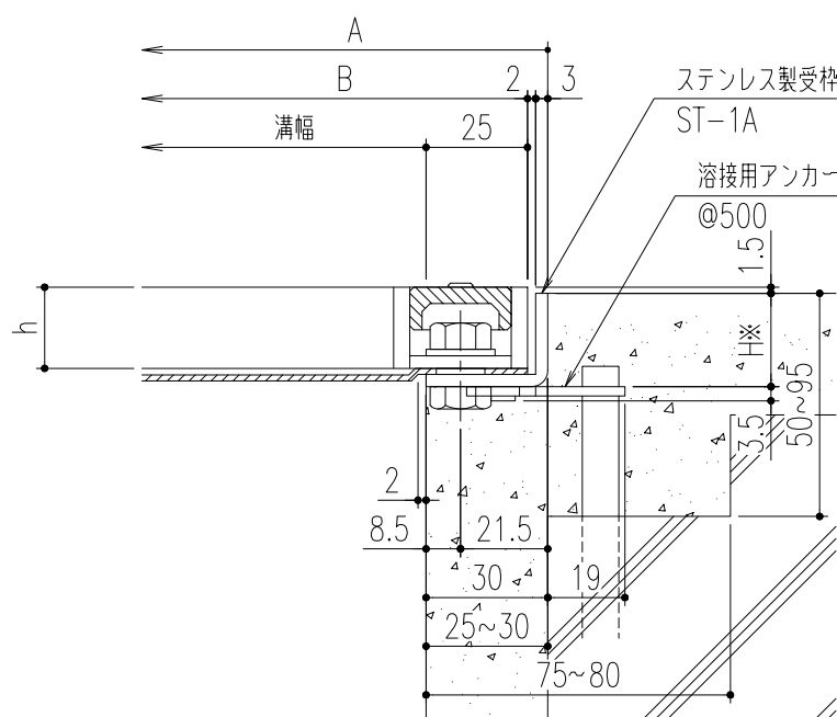
断面詳細図
