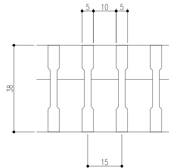
へアリングバー-断面詳細図
